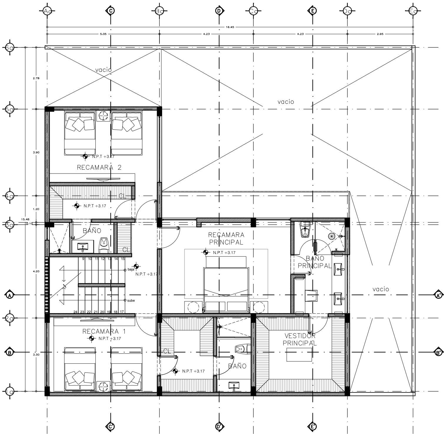
PLANTA ALTA CASAS 5-6
