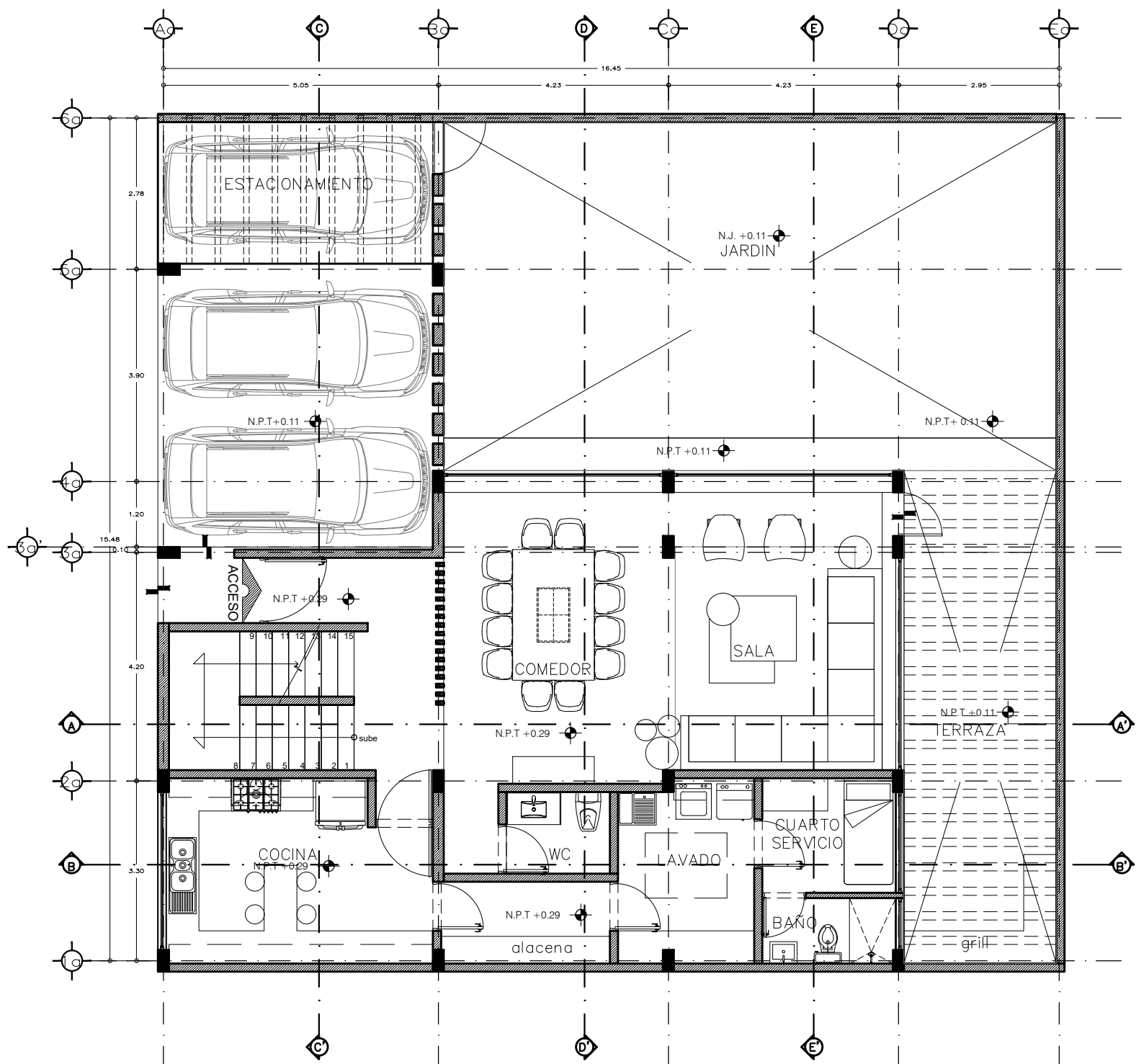
PLANTA BAJA CASAS 5-6
